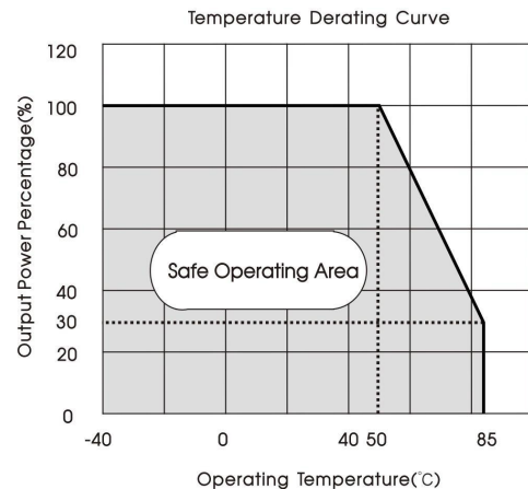
Fig.2 K78U24-300R3 (Vin≥60V)
