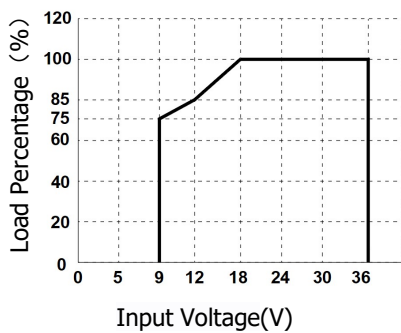
Load VS Vin (24V)
