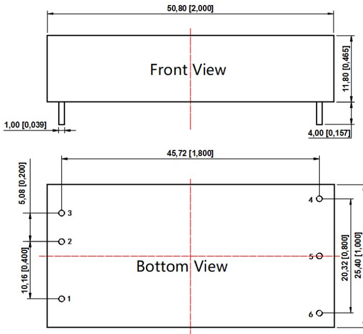
ATB_LD-60WR3 Dimensions
